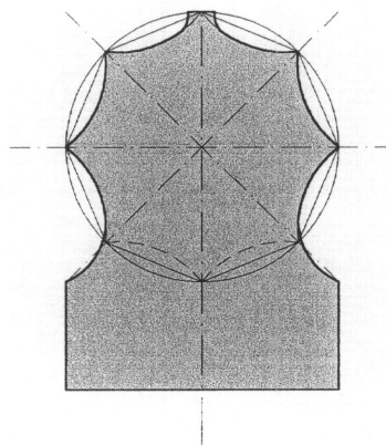
PERPIAÑO HELICOIDAL DE ARISTA VIVA.
