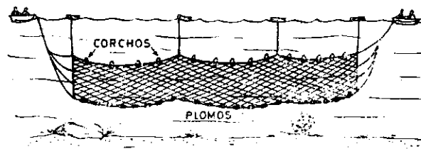
Fig. 6.—Sadinal de enmalle.
