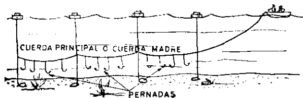
Fig. 8.—Palangre de fondo.
