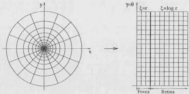
Figura 3.4: El sensor log-polar CMOS de IMEC
