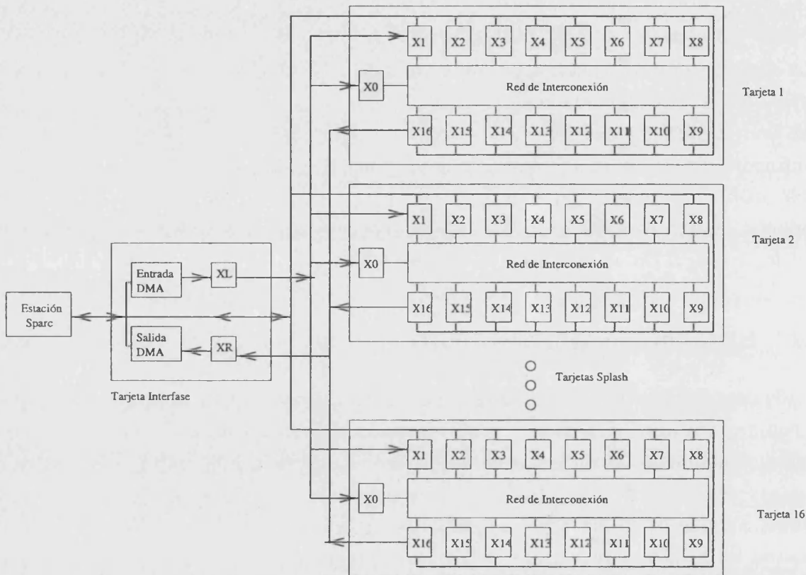
Figura 2.3: Arquitectura del sistema Splash-2
