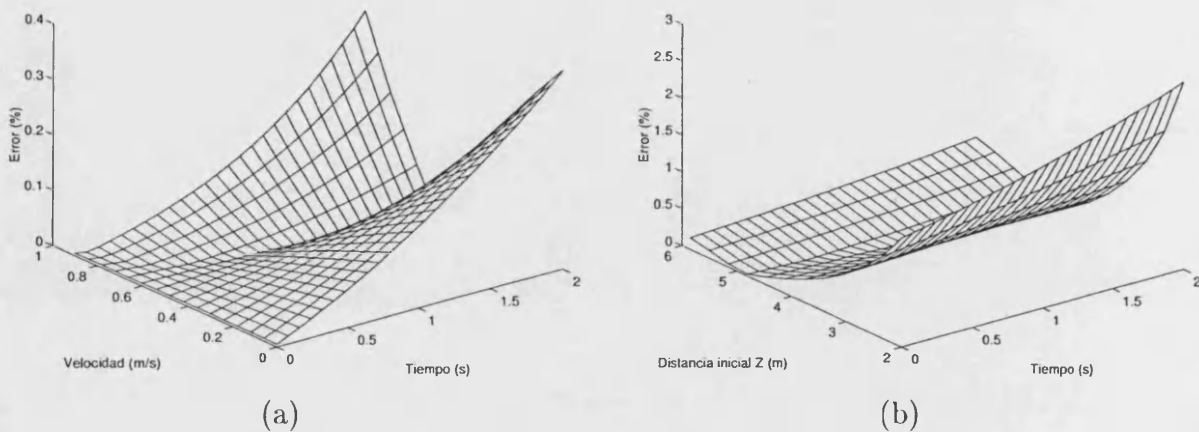
Figura 8.5: Error en el algoritmo de detección de movimiento en función de la velocidad (a) y la distancia (b)
