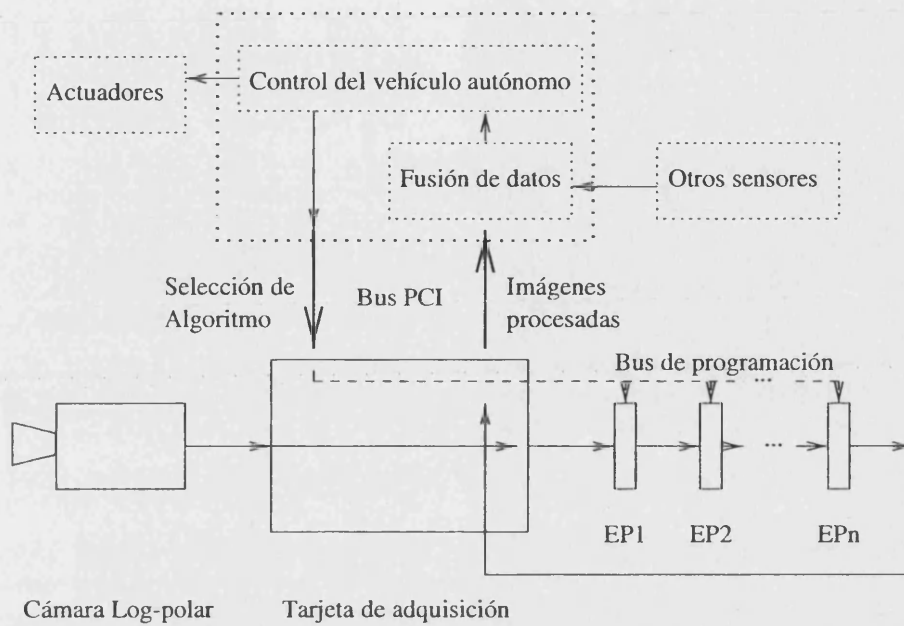
Figura 4.1: Flujo de datos a través del cauce segmentado
