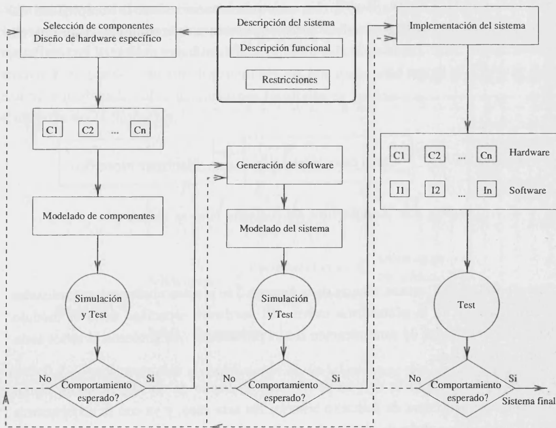
Figura 5.2: El ciclo de diseño clásico
