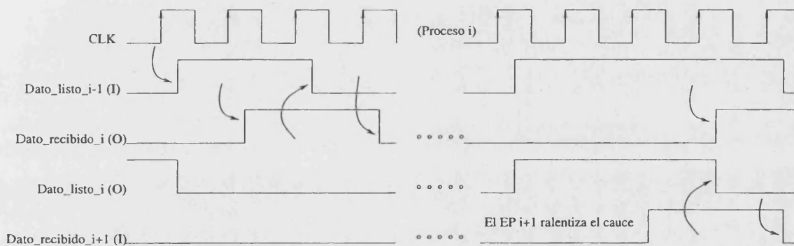
Figura 4.2: Transmisión de datos a través del cauce segmentado
