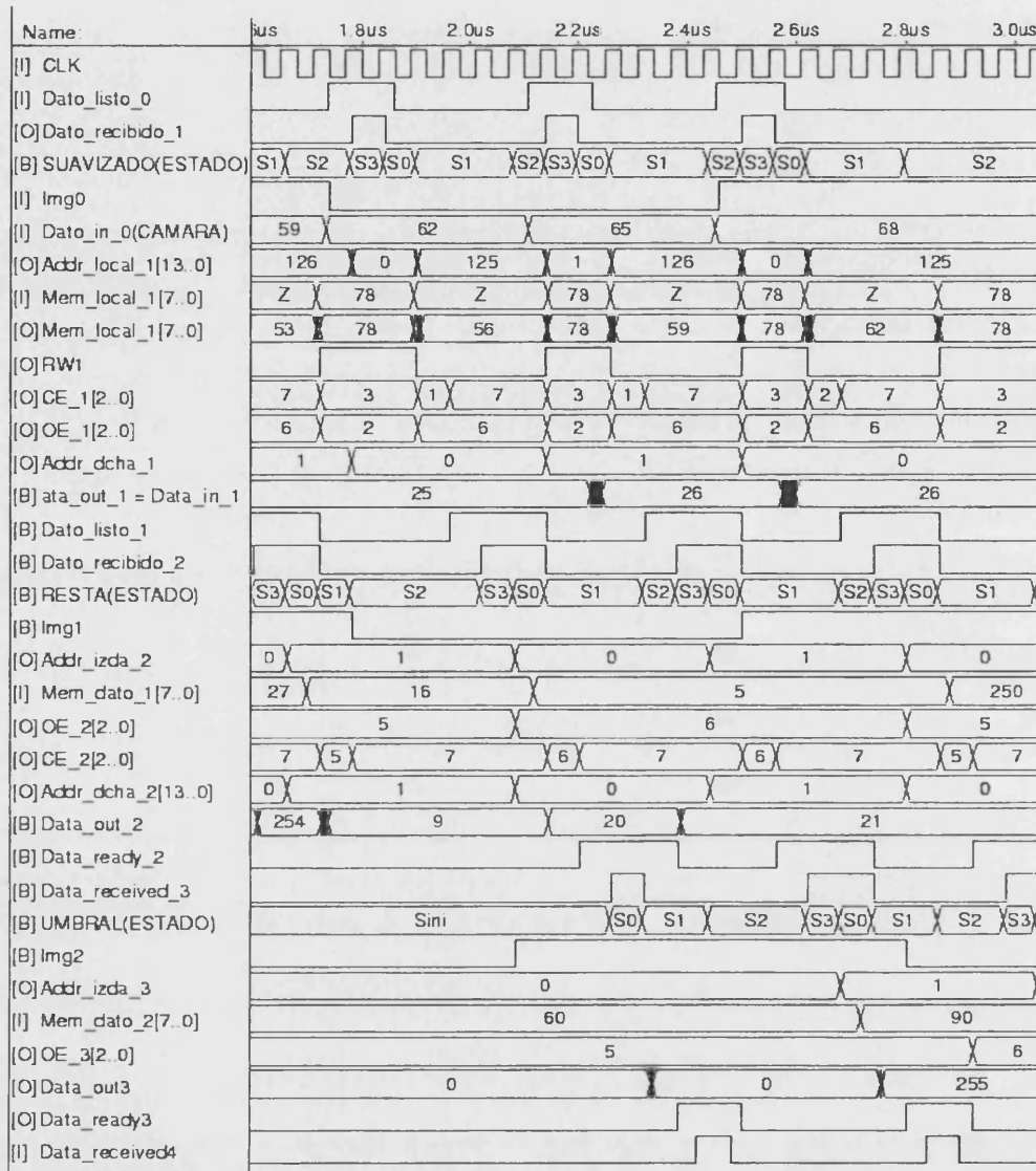
Figura 6.3: Simulación del algoritmo de detección de movimiento con imágenes de 2 bits
