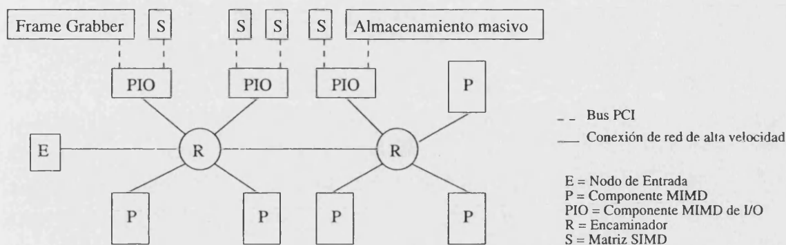
Figura 2.2: Arquitectura CC/IPP
