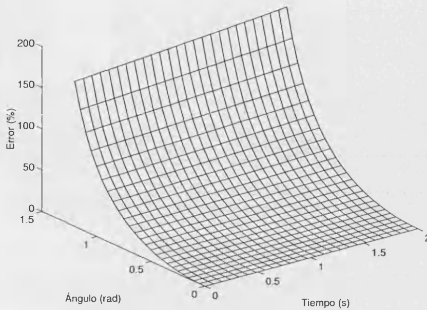
Figura 8.6: Error en el cálculo del tiempo al impacto función del ángulo
