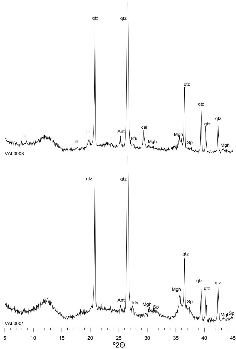
Figura 7. Grup A. Difractograma del individu VAL0008 (dalt) representant la fàbrica 1 i VAL0001 (inferior) representant la fàbrica 2:ill: illita-muscovita, qtz:quars, Ant: anatasa, kfs: feldspats alcalins, cal: calcita, Mgh: maghemita, Sp: espinel·la
