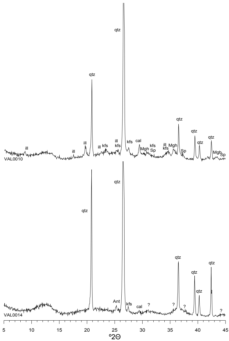
Figura 10. Difractograma del individu VAL0010 (dalt) representant el grup C i VAL0014 (inferior) representant el grup D :ill: illita-muscovita, qtz:quars, Ant: anatasa, kfs: feldspats alcalins, cal: calcita, Mgh: maghemita, Sp: espinel·la
