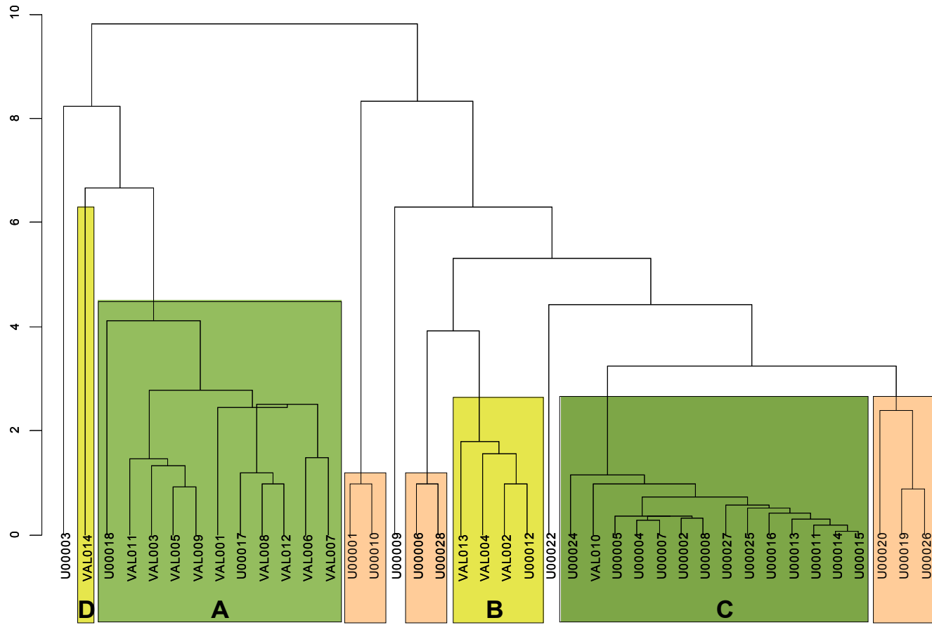
Figura 5. Dendrograma resultant de l'anàlisi d'agrupament utilitzant la distància euclidiana al quadrat i el procés aglomeratiu del centroide per la subcomposició Fe_2O_3 (com Fe total), Al_2O_3 , MnO, TiO_2 , MgO, CaO, Na_2O , K_2O , Ba, Rb, Th, Nb, Zr, Y, Sr, Ce, Ga, V, Zn, Ni i Cr transformats en logaritmes de raons utilitzant el SiO_2 , com a divisor. Destacats en requadres de colors verd i groc, els grups on es troben les mostres de València analitzades. Amb la sigla UXXXXX els individus del grup de contrast. En requadres rosa, grups formats només per individus del grup de contrast
