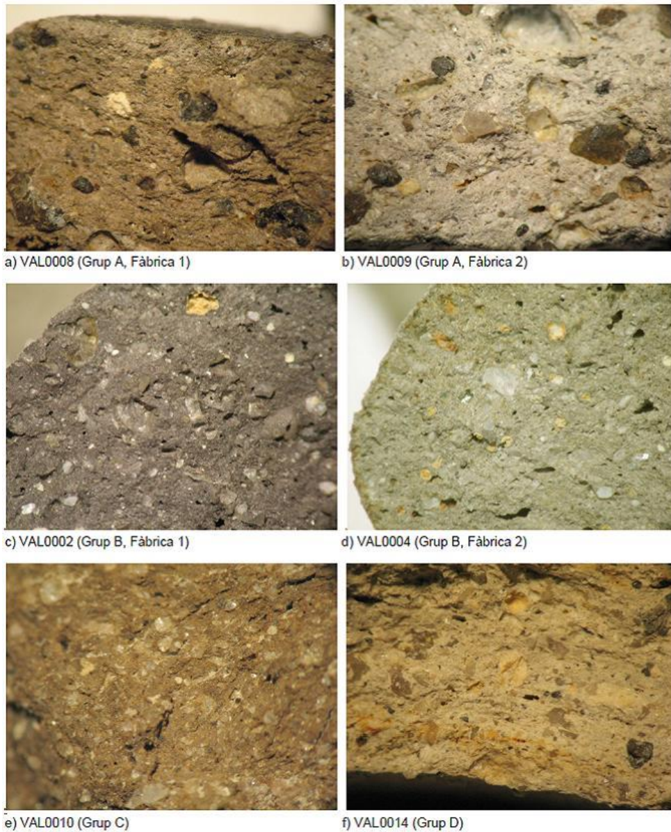
Figura 265: Microfotografies per lupa binocular a 25x de diferents mostres procedents de Valentia .
