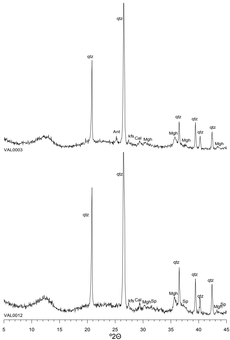
Figura 8. Grup A. Difractograma del individu VAL0003 (dalt) representant la fàbrica 3 i VAL0012 (inferior) representant la fàbrica 4: qtz:quars, Ant: anatasa, kfs: feldspats alcalins, cal: calcita, Mgh: maghemita, Sp: espinel·la
