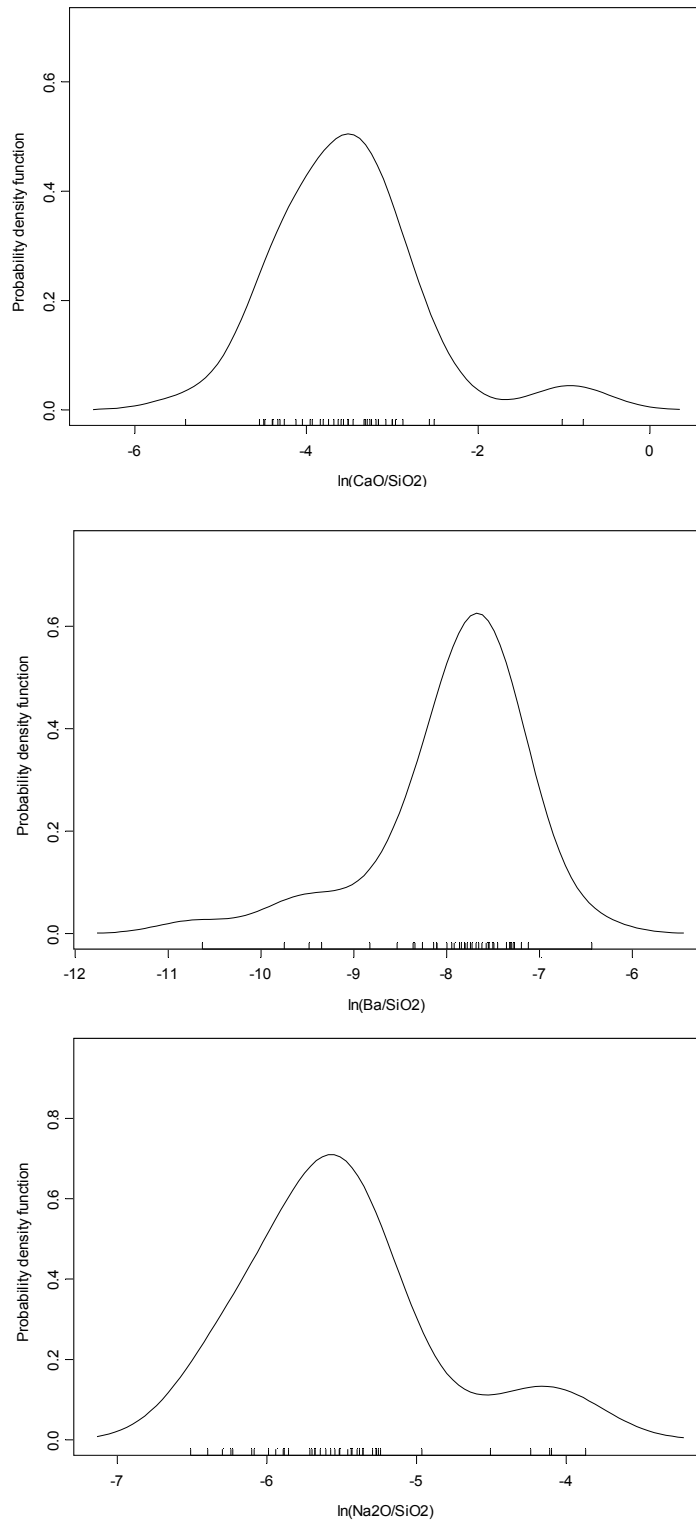
Figura2. Estimacions de densitat per Kernel dels \ln(\text{CaO}/\text{SiO}_2) , dalt; \ln(\text{Ba}/\text{SiO}_2) , centre; i \ln(\text{Na}_2\text{O}/\text{SiO}_2) , baix
