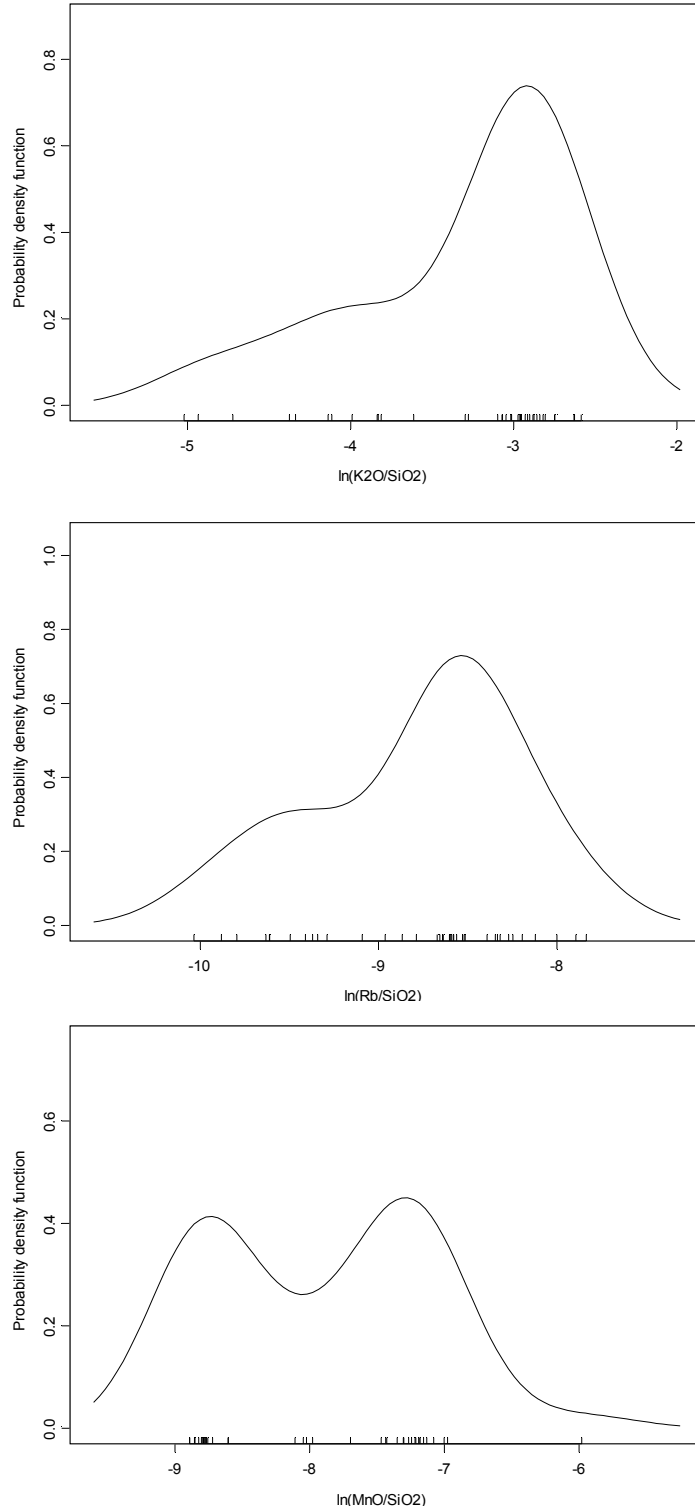
Figura 2 (Continuació). Estimacions de densitat per Kernel dels \ln(K_2O/SiO_2) , dalt; \ln(Rb/SiO_2) , centre; i \ln(MnO/SiO_2) , baix
