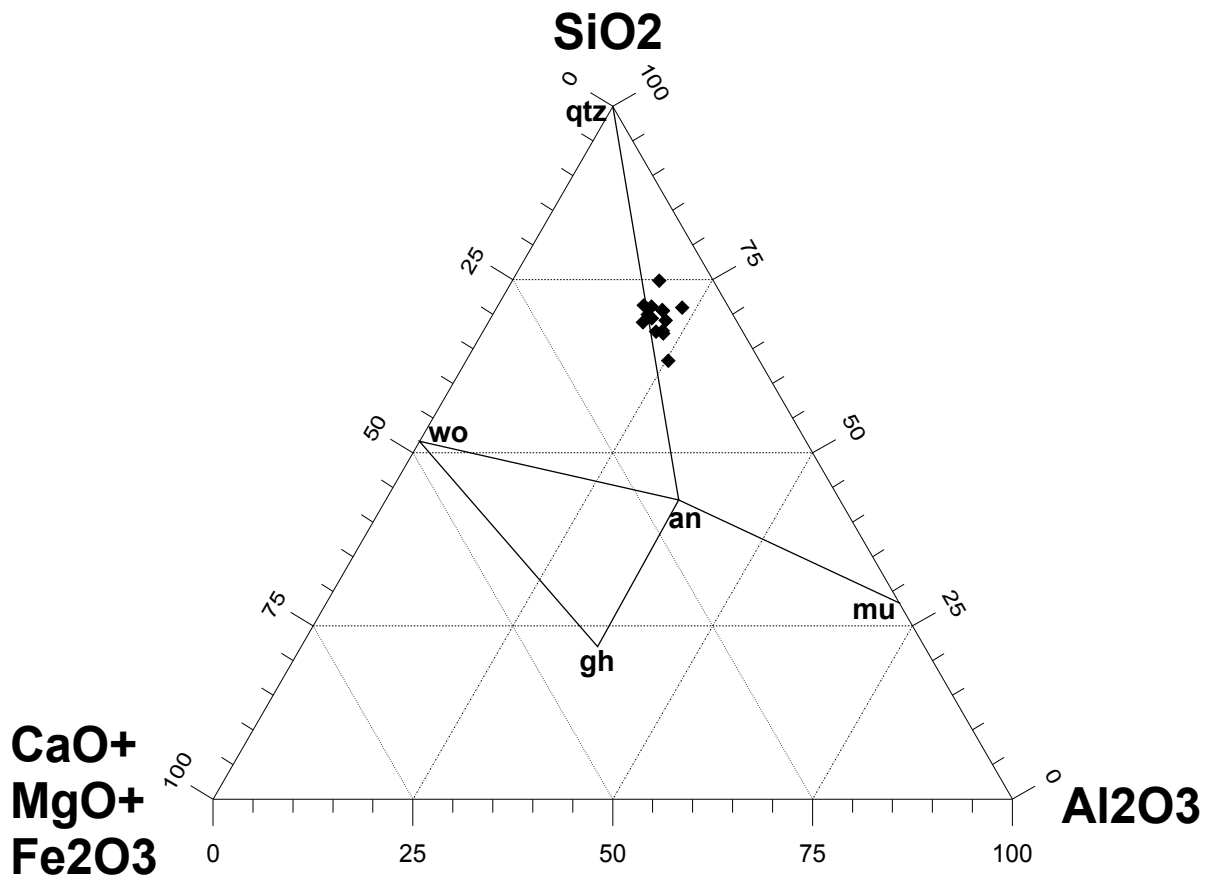
iO 2 -Al 2 O 2 -CaO+MgO+Fe 2 O 3 (triangle ceràmic) amb la situació dels individus analitzats. qtz: quars; wo: wollastonita; an: anortita; mu: mullita; gh: gehlenita
