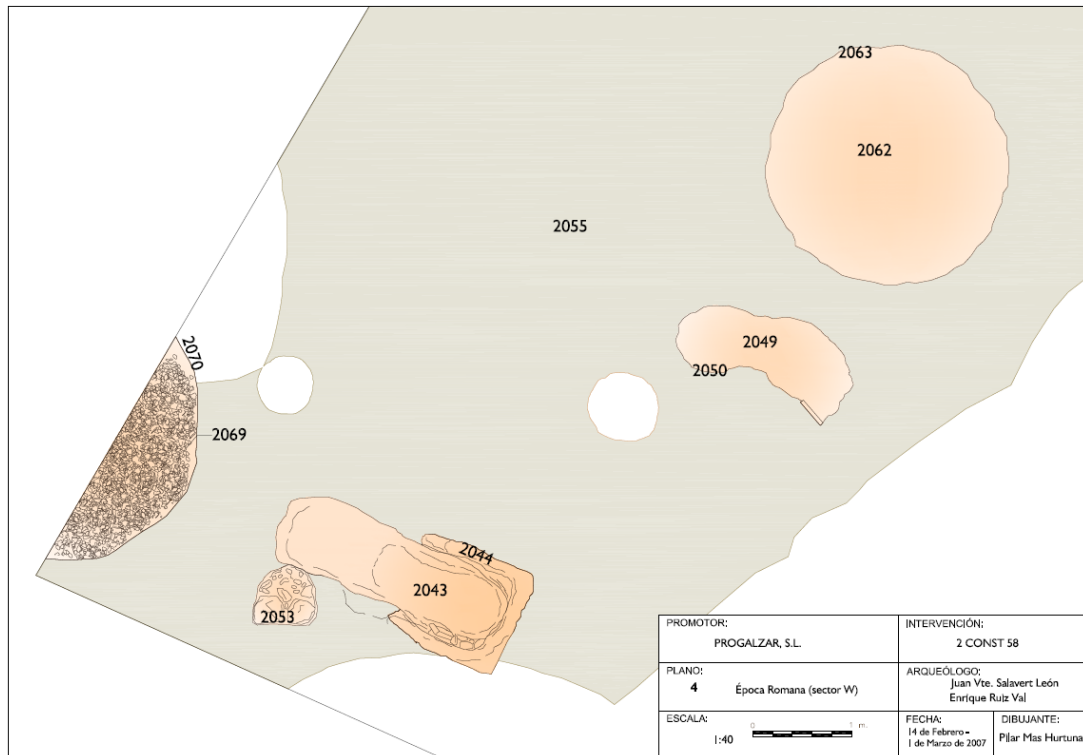
Figura 71: Nivells romans de l'excavació d'Avinguda de la Constitució núm. 58 on s'observa la planta del forn de ceràmica comuna i de la fossa amb el rebuig d'una fornada fallida.
