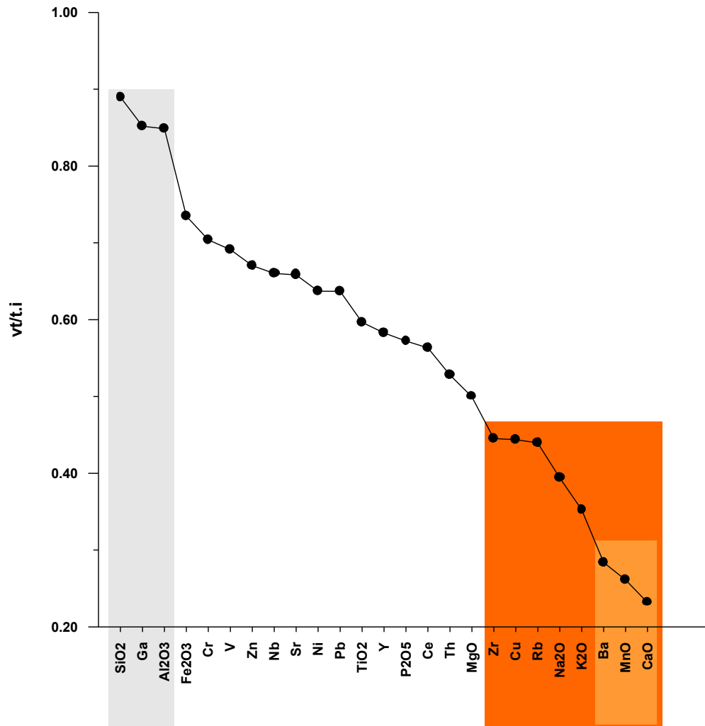
Figura 1. Diagrama bivariant amb els components retinguts per a l'anàlisi ordenats per rang descendent, en abscisses, i el valor vt/t.i, en ordenades, que presenten en la matriu de variació composicional
