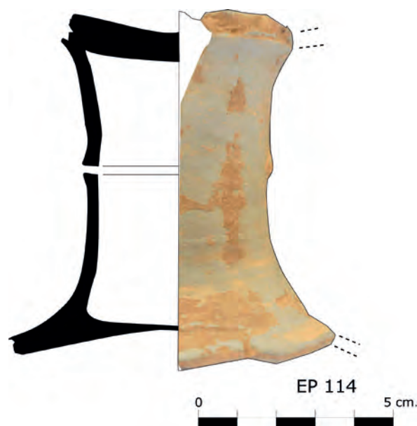
Figura 11. Diábolo/carrete.
