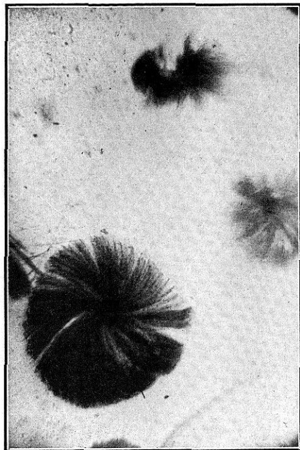
FIG. 19. Yoduro de narceína
