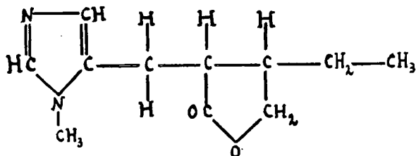
Pilocarpina
