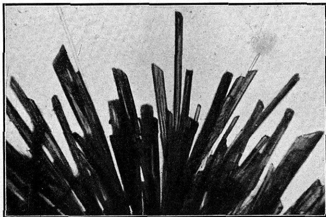
FIG. 21. Yoduro de quinidina
