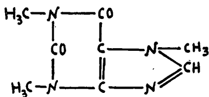
Cafeína
