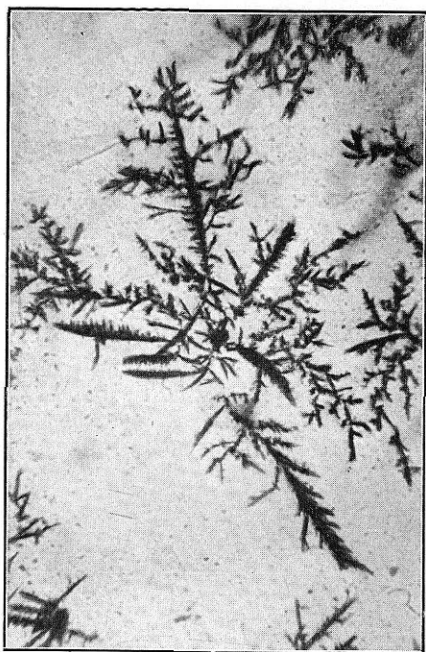
FIG. 46. Bromoaurato de hidrastinina
