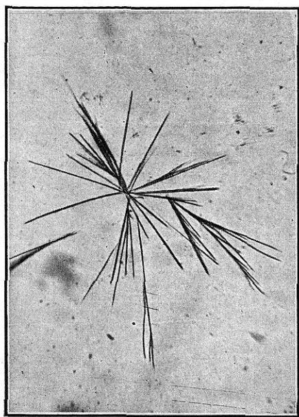
FIG. 13. Yoduro de estriquina
