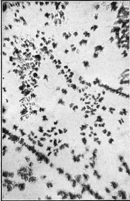
FIG. 33. Yodocadmiato de papaverina
