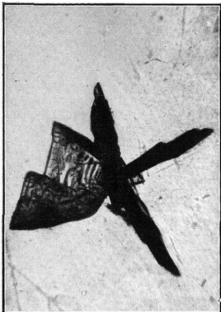
FIG. 9. Yoduro de cinconina Mayor concentración
