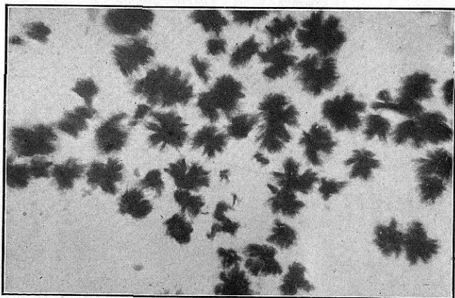
FIG. 52. Bromoaurato de teobromina
