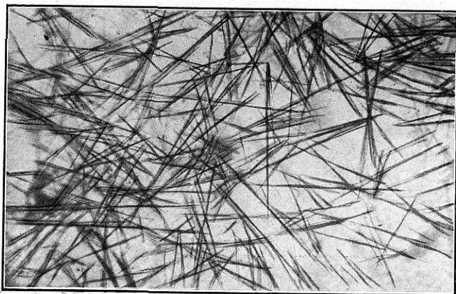
FIG. 50. Bromoaurato de pilocarpina
