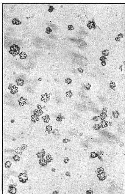
FIG. 38. Cromato de estricnina
