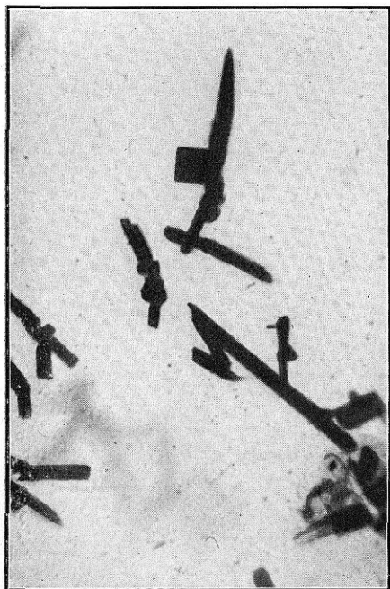
FIG. 11. Yoduro de escopolamina
