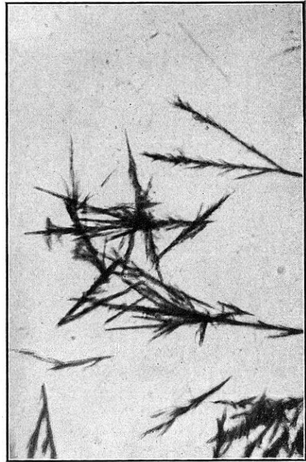
FIG. 30. Yodocadmiato de estriquina
