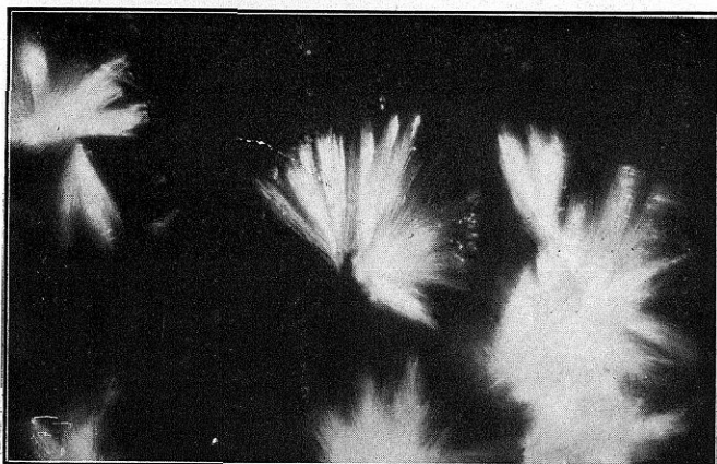
FIG. 51. Bromoaurato de quinidina
