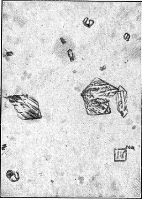
FIG. 1. Yoduro de aconitina
