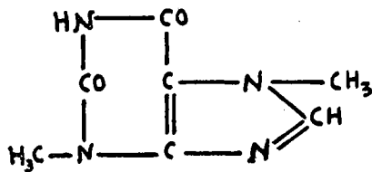
Teobromina
