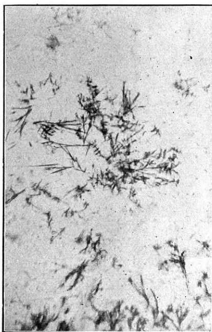
FIG. 36. Cromato de apomorfină
