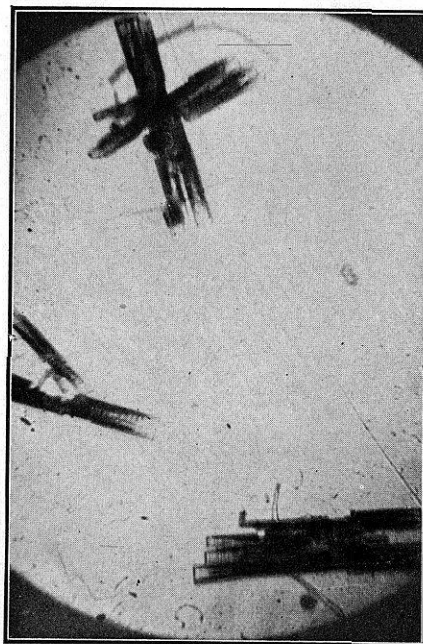
FIG. 56. Bromato de escopolamina
