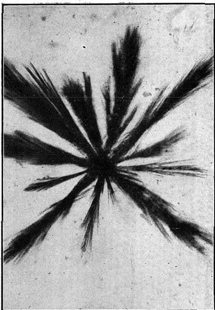
FIG. 10. Yoduro de codeína
