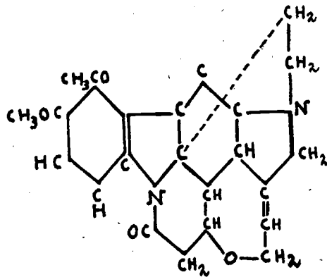
Brucina
