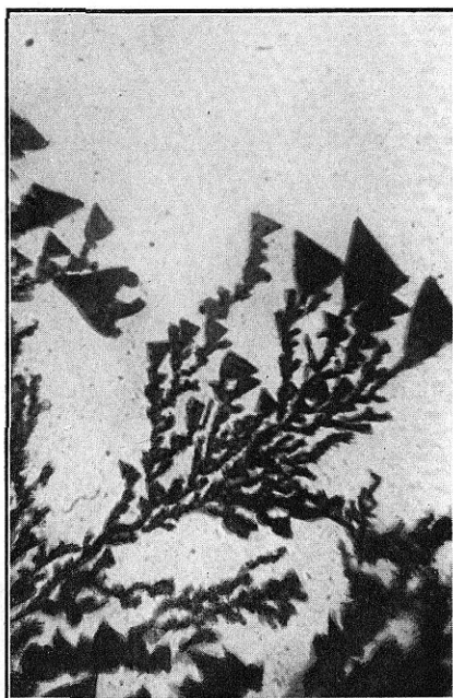
FIG. 47. Bromoaurato de hiosciamina
