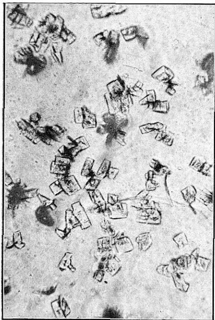
FIG. 25. Yodocadmiato de aconitina
