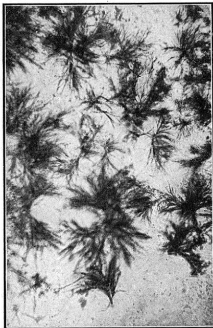
FIG. 40. Cromato de lobelina
