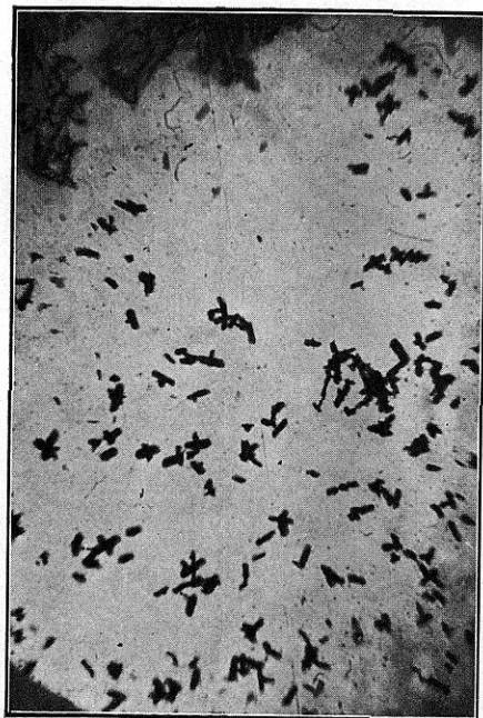
FIG. 55. Bromato de cafeína
