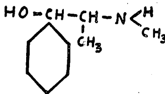
Efedrina
