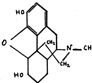
Morfina
