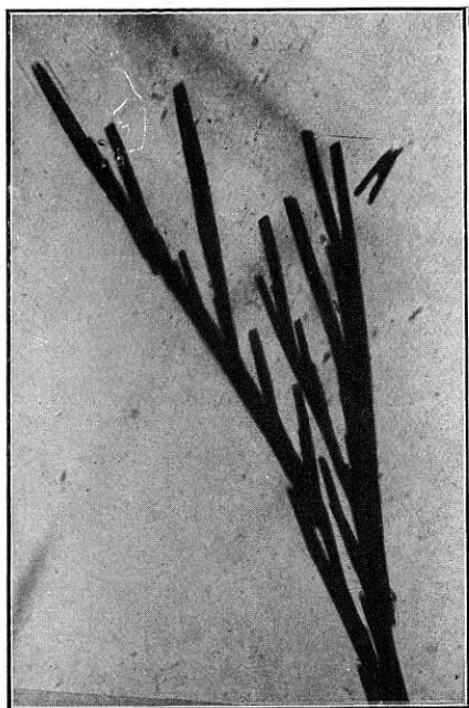
FIG. 39. Cromato de hidrastinina
