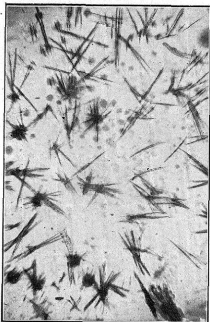
FIG. 64. Narcotina + Piridina
