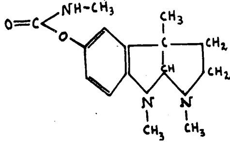
Eserina
