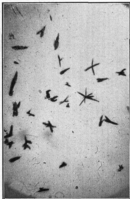
FIG. 57. Bromato de hiosciamina
