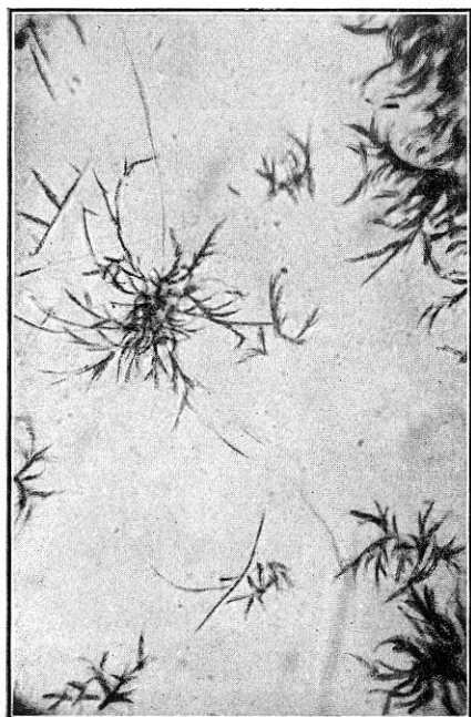
FIG. 37. Cromato de cinchonidina
