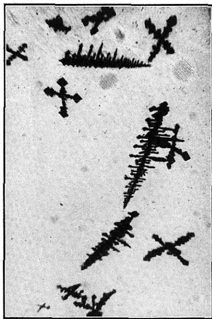
FIG. 20. Yoduro de pilocarpina
