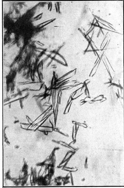
FIG. 34. Yodocadmiato de quinina
