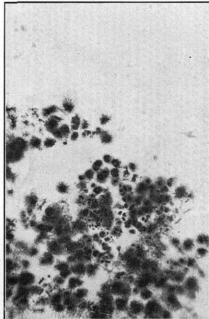
FIG. 4. Yoduro de berberina
