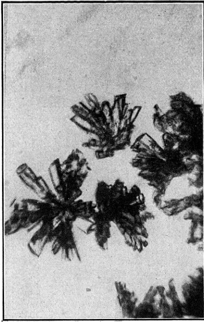
FIG. 29. Yodocadmiato de codeína
