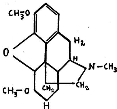
Tebaina
