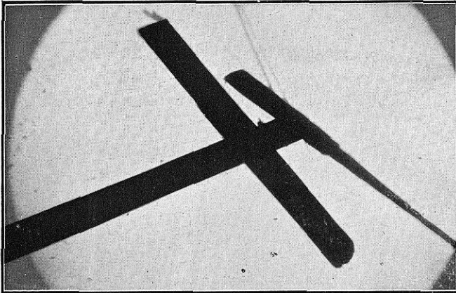
FIG. 24. Yoduro de teobromina
