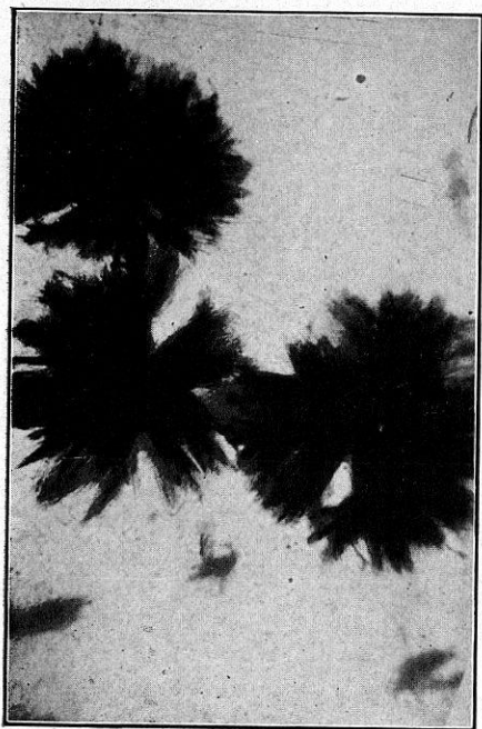
FIG. 68. Yodoaurato de esparteína
