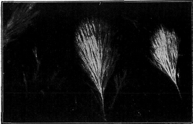
FIG. 61. Bromato de quinidina Aumento 4 diámetros
