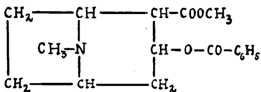
Cocaína
