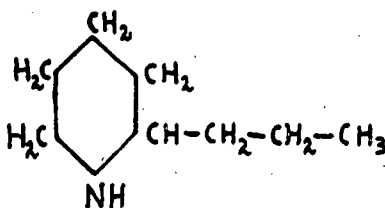
Cicutina
