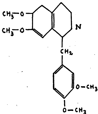
Papaverina
