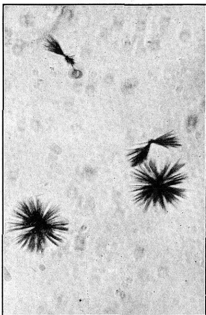
FIG. 26. Yodocadmiato de berberina
