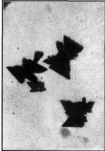
FIG. 6. Yoduro de cafeína
