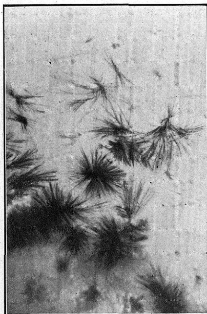
FIG. 59. Bromato de morfina
