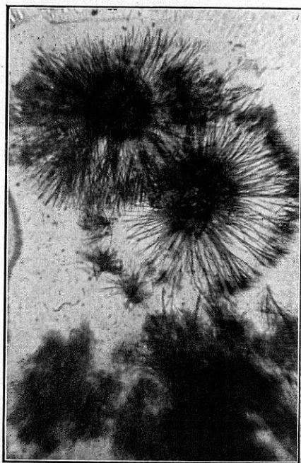
FIG. 69. Picrolonato de estircina
