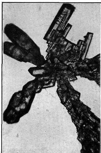
FIG. 28. Yodocadmiato de cinconina
