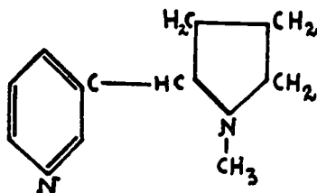
Nicotina
