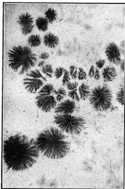
FIG. 35. Cromato de aconitina
