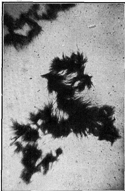
FIG. 15. Yoduro de hiosciamina
