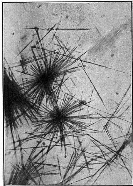
FIG. 32. Yodocadmiato de morfina
