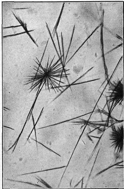
FIG. 63. Bromato de berberina
