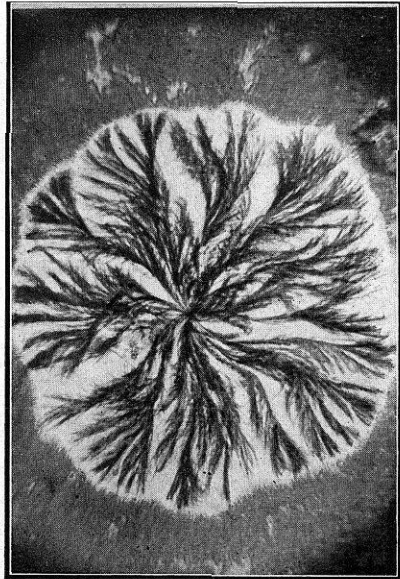
FIG. 8. Yoduro de cinconina
