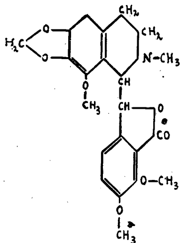
Narcotina
