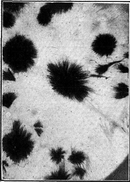
FIG. 5. Yoduro de brucina
