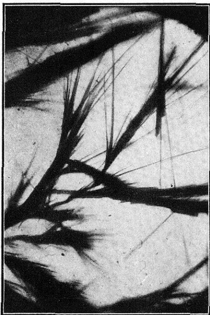
FIG. 17. Yoduro de mescalina
