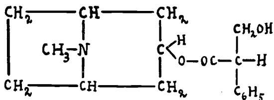
Atropina
