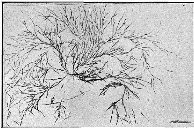
FIG. 16. Yoduro de mescalina Aumento 4 diámetros
