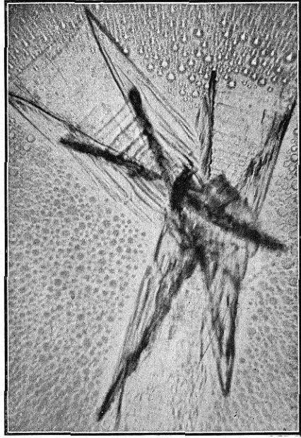
FIG. 23. Yoduro de quinina Mayor concentración
