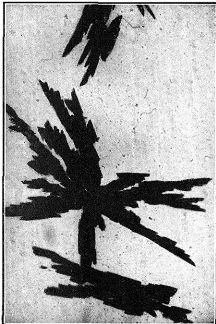
FIG. 18. Yoduro de morfina
