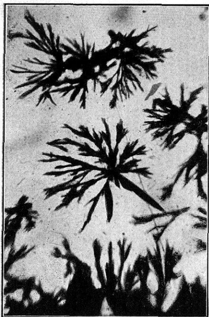
FIG. 42. Bromoaurato de arecolina
