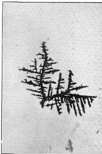
FIG. 49. Bromoaurato de peletierina
