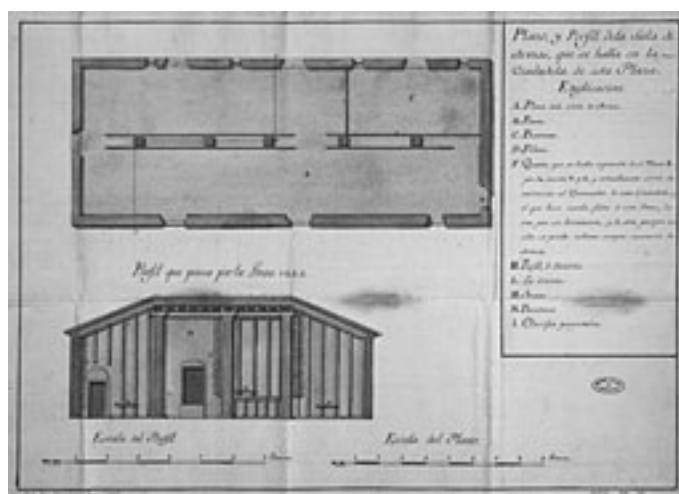
Fig. 5. Plano y perfil de la Sala de Armas... AGS, Mapas, Planos y Dibujos, 54/016.
