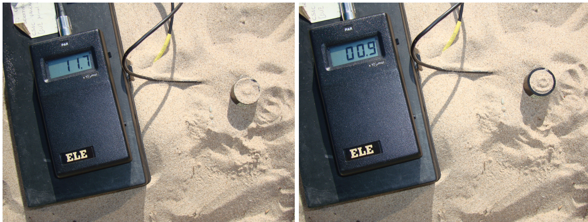
Fig. 2.18: Medición de la radiación fotosintéticamente activa (PAR)
