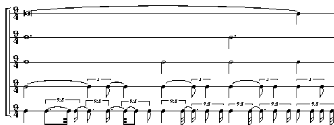
Schéma 8b : Gamelan ternaire.
