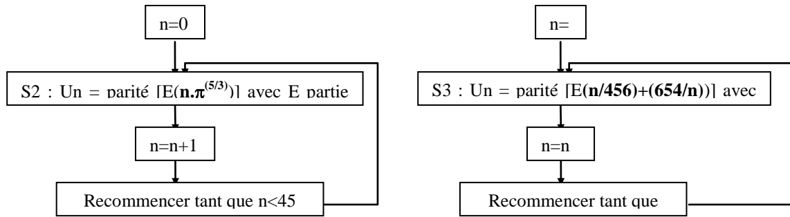
Schéma 6b et 6c : algorithmes d'engendrement des séries S2 et S3
