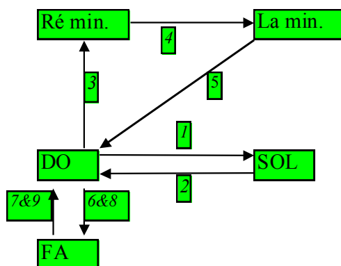
Schéma 1 : Modélisation par André Riotte du parcours harmonique de l' Invention n°1 BWV 772 de J.-S. Bach
