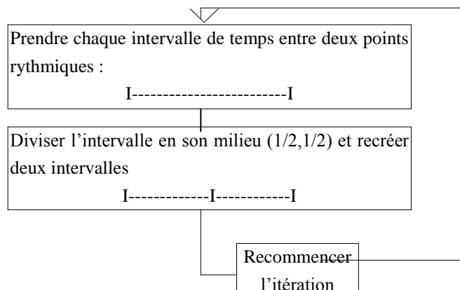
Schéma 7a : algorithme générateur du Gamelan binaire
