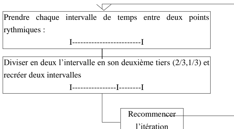
Schéma 8a : algorithme générateur du Gamelan ternaire
