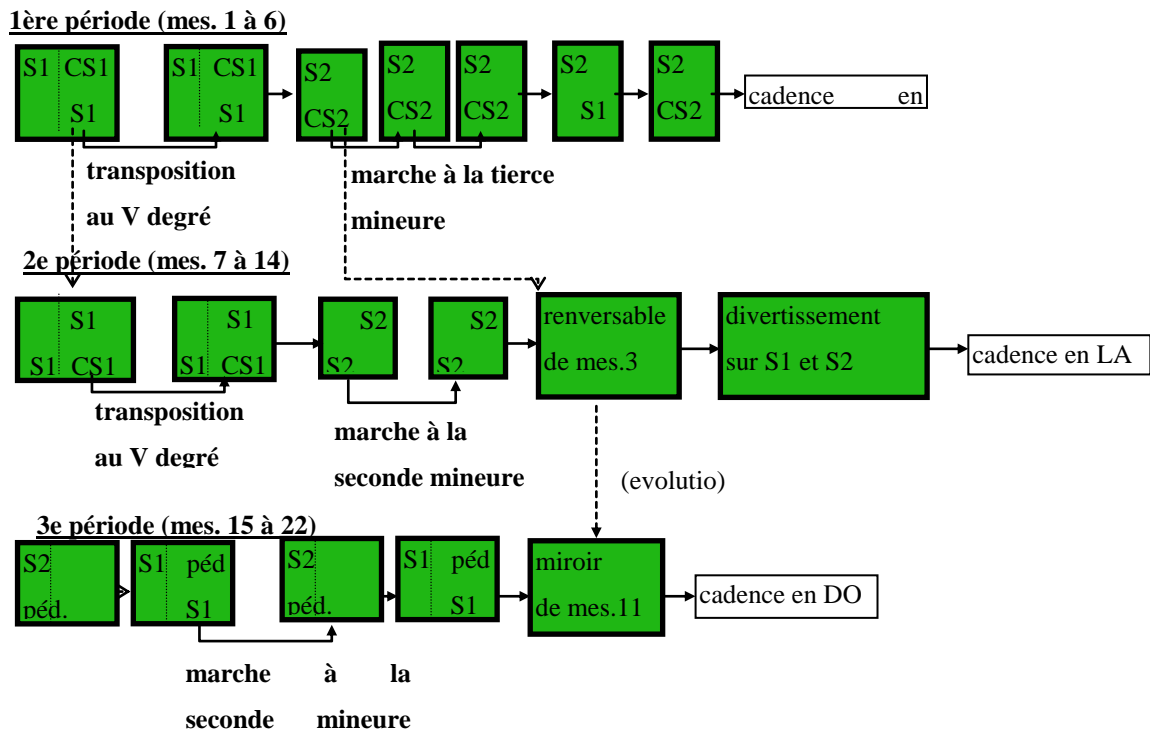
Schéma 2 : modélisation par automate des différents motifs de l'Invention n°1 BWV 772 de J.-S. Bach (S1 : sujet 1; CS1 : contre-sujet 1)
