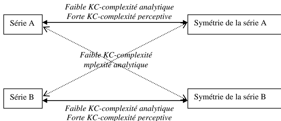
Schéma 11: non -bijection des complexités aperceptives et grammatologiques
