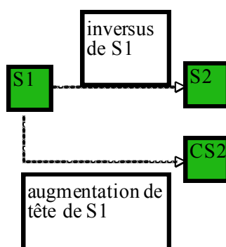
Schéma 3: modélisation par automate des relations entre motifs (Invention n°1 à 2 voix BWV 772 de J.S. Bach)
