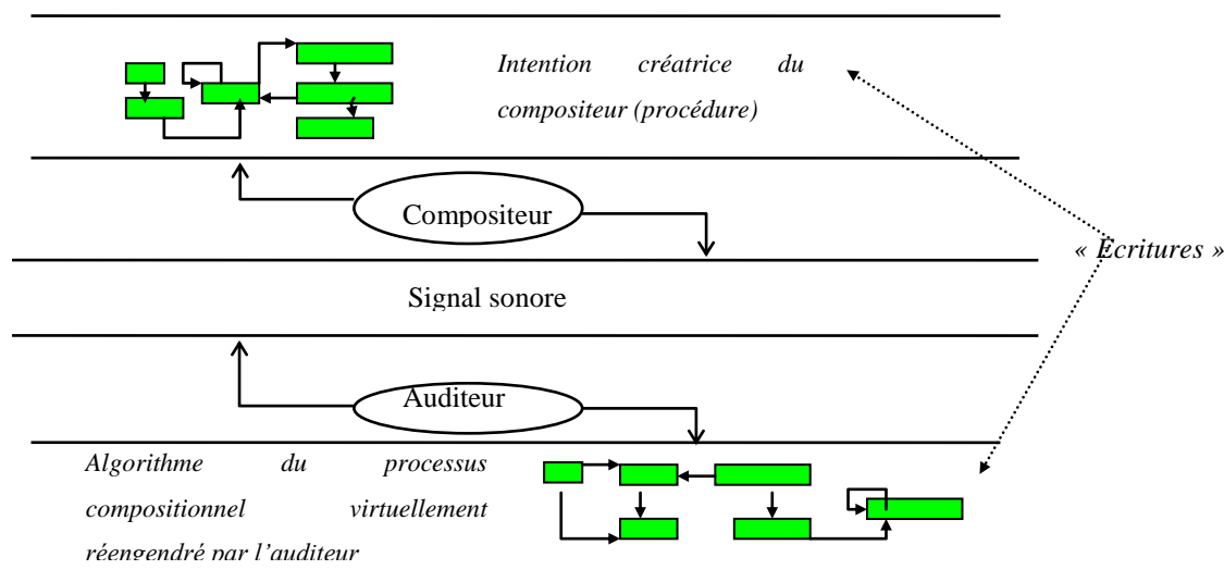
Schéma 4: l'aperception comme réécriture
