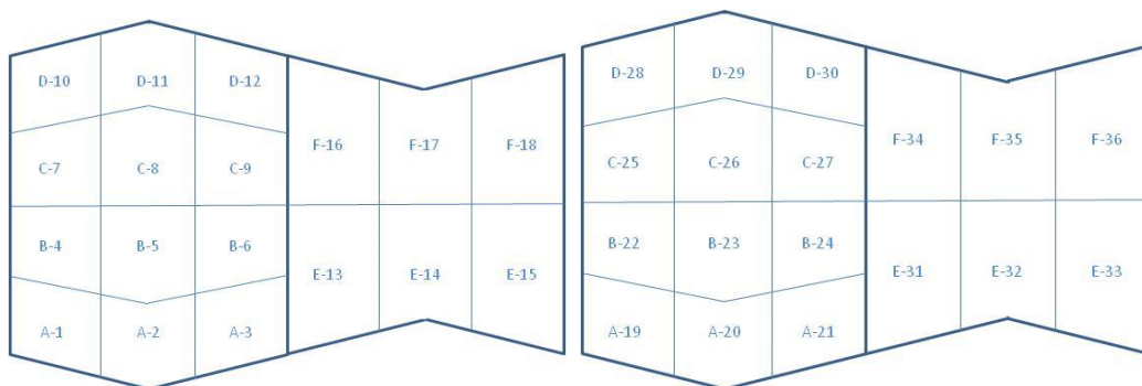
Figura 7.8. Segmentación virtual 3 del conducto de ventilación para la medida por tasa de dosis
