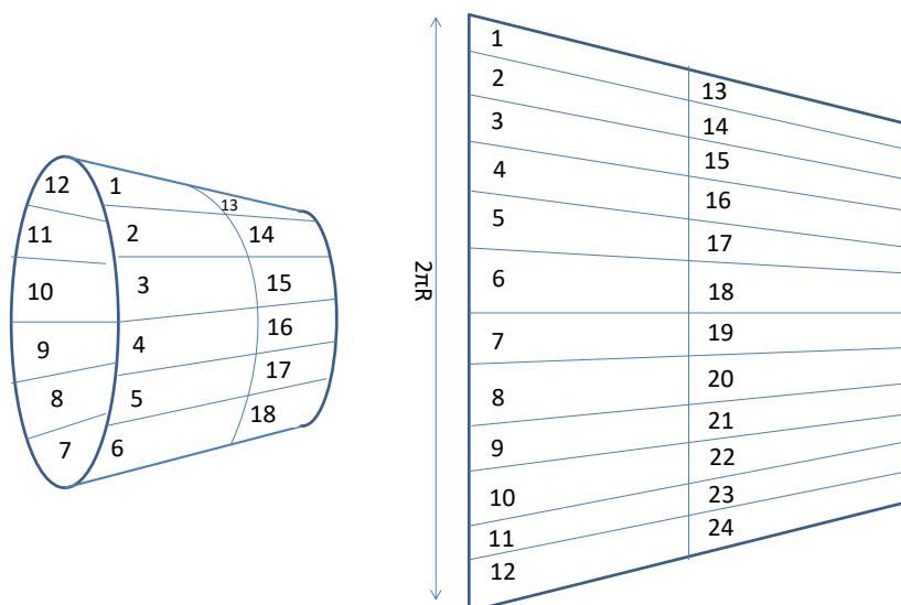
Figura 7.2. Segmentación virtual llevada a cabo para el carrete de la rama intermedia
