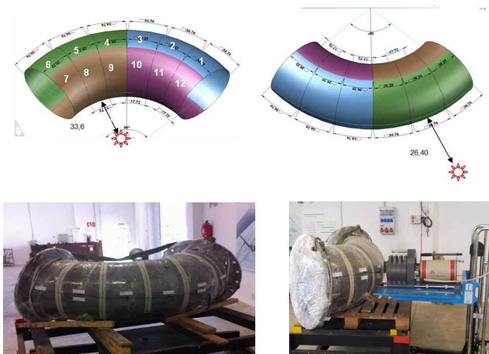
Figura 7.10. Segmentación virtual 2 del conducto de ventilación para la medida por espectrometría Gamma. Imagen real final del conducto y medida con equipo ISOCS.
