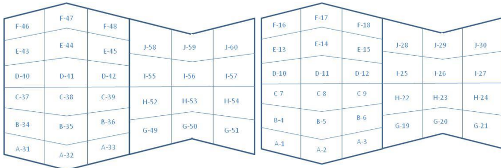
Figura 7.7. Segmentación virtual 2 del conducto de ventilación para la medida por tasa de dosis.
