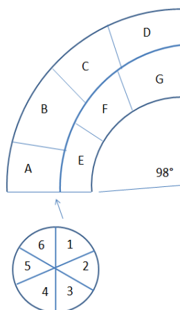
Figura 7.5. Segmentación virtual llevada a cabo en el conducto de ventilación para medida por tasa de dosis.
