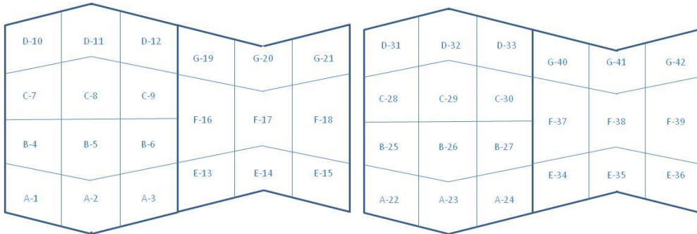
Figura 7.6. Segmentación virtual 1 del conducto de ventilación para la medida por tasa de dosis.
