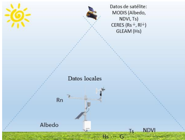
Figura 7. Esquema de un sistema natural con las variables que determinan ET_p y ET_r .
