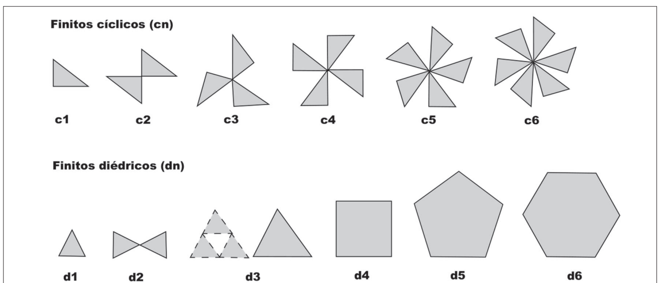
Fig. 3.19: Motivos finitos contruidos por rotación o cíclicos (cn) y diédricos (dn). Elaboración propia a partir de la Fig. 21 de Washburn, 2018.
