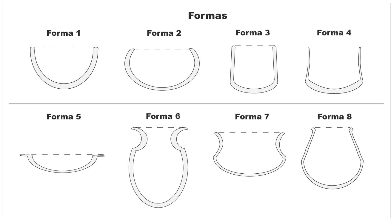
Fig. A.5: Formas 1 a 8. En línea discontinua se representa el Db.
