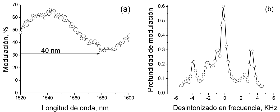
FIGURA 7. (a) Profundidad de modulación en función de la longitud de onda. (b) Profundidad de modulación en función del desintonizado en frecuencia ( \Delta f_a ) manteniendo fijos la longitud de onda resonante en 1545 nm y el voltaje de RF en 10.2 V. La frecuencia central en la Fig. 4(b) es 1.1565 MHz.
