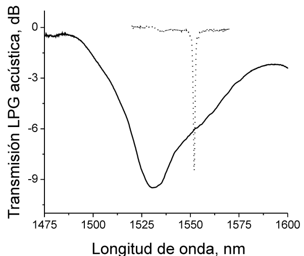
FIGURA 5. Transmisión espectral para una LPG inducida acústicamente en una fibra estrechada biconica de 70 \mu\text{m} (línea sólida). La línea punteada representa la transmisión espectral para una fibra estándar sin estrechar. Las frecuencia acústica se fijaron en 1.014 MHz y 2.37315 MHz, respectivamente.
