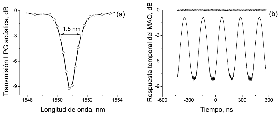
FIGURA 2. (a) Transmisión espectral de la LPG inducida acústicamente en el MAO alrededor de la resonancia localizada en 1550.8 nm. (b) Traza del osciloscopio que corresponde a la transmisión temporal del MAO grabada a la longitud de onda de resonancia; el nivel de referencia es la línea continua correspondiente a 0 dB de transmisión. En ambos casos f_a = 2.37315 \text{ MHz} y V_{DP} = 18 \text{ V} .
