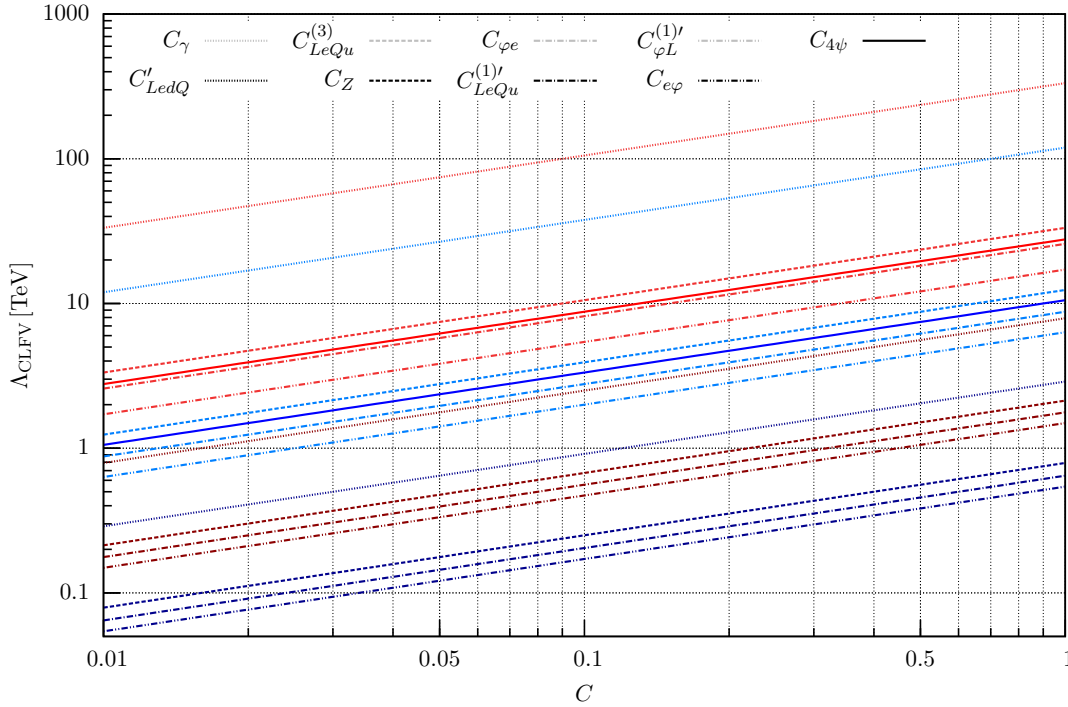
FIGURE 7.1: Restriccions sobre \Lambda_{\text{CLFV}} respecte als valors dels WCs, basades en els límits actuals de Belle (tons en blau) i en els límits esperats de Belle II (tons en roig) i donades al 99.8% nivell de confiança. Els WCs amb quatre fermions es representen en conjunt com a C_{4\psi} . Per a un conjunt donat de límits (distinguits per tons blaus i rojos), els tons més clars corresponen als WCs llistats en la fila de dalt de la llegenda (sense contar el comú als WCs amb 4 fermions C_{4\psi} ), i els tons més obscurs corresponen als WCs de la fila de baix.
