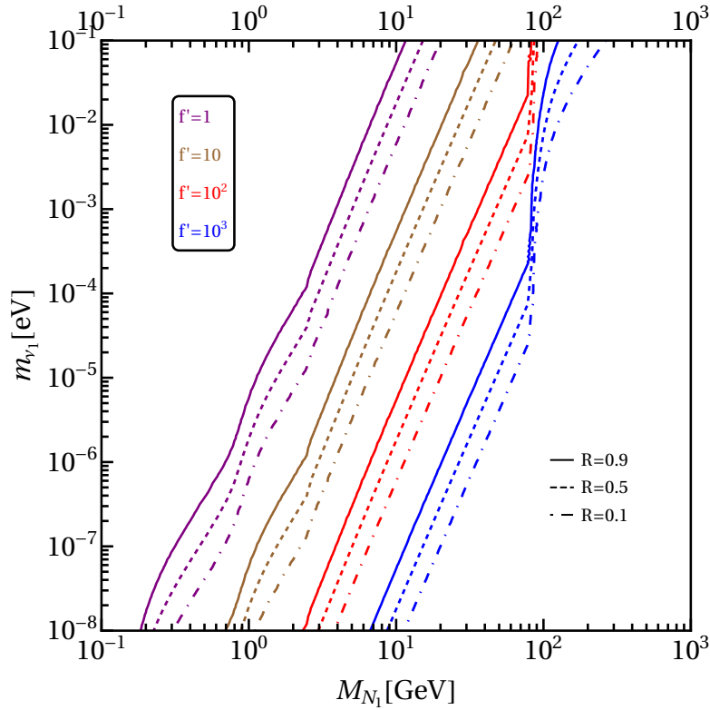
FIGURE 7.3: Línies m_{\nu_1}-M_{N_1} corresponents a un valor específic de R_{\ell\ell} i f' . Per a cada color, les tres línies corresponen a valors de R_{\ell\ell} = 0.9, 0.5 i 0.1 d'esquerra a dreta.
